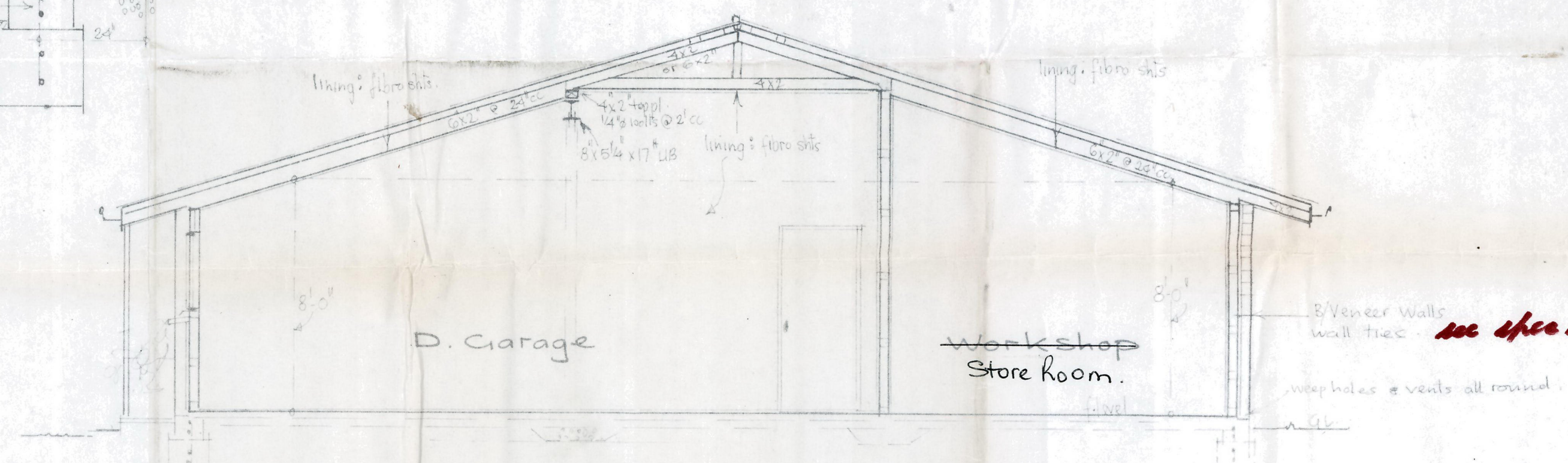
~ Section 'BB' ~
